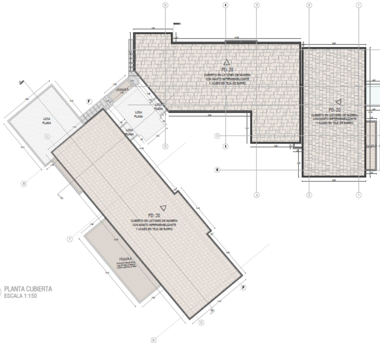
PLANTA DE CUBIERTA
